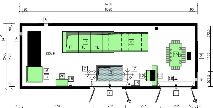
PIANTA CABINA
