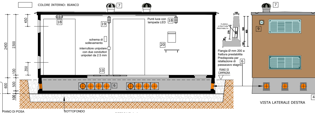
SEZIONE A-A
