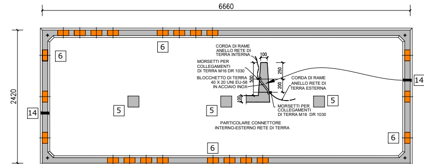
PIANTA VASCA DI FONDAZIONE
